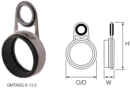
GMTAガイド (テレガイド) 口金接着型。機上物竿用
