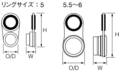
GMTMガイド (テレガイド) 遊動型。機上物竿用
